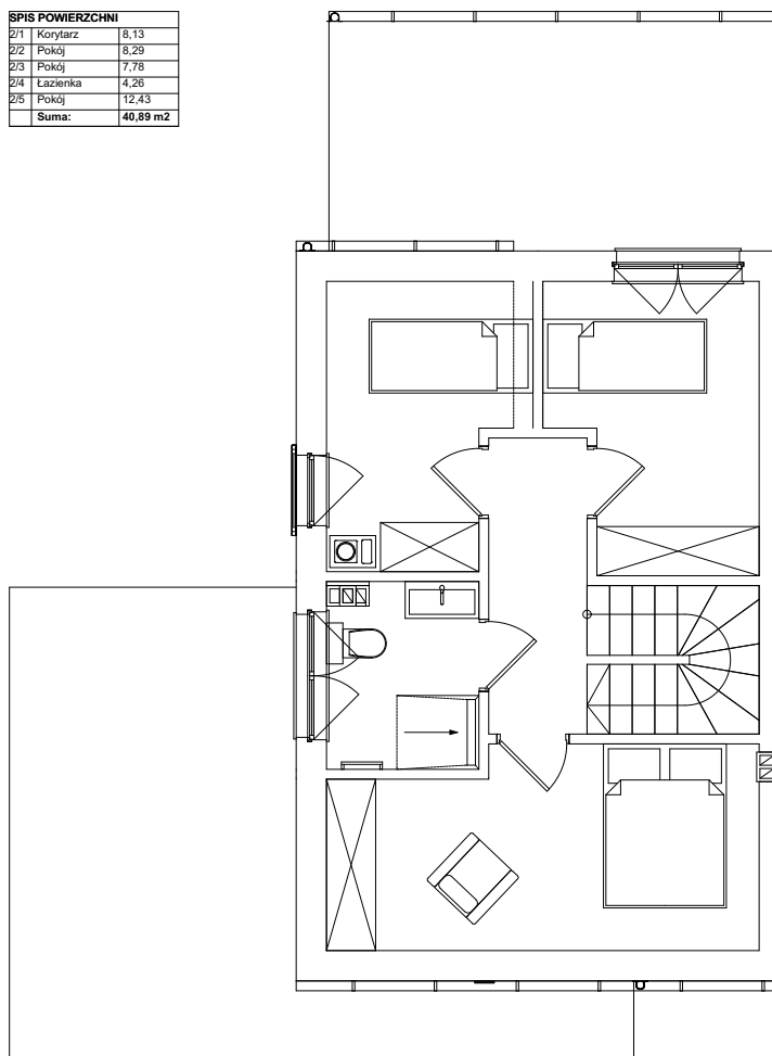
PODDASZE RZUT
